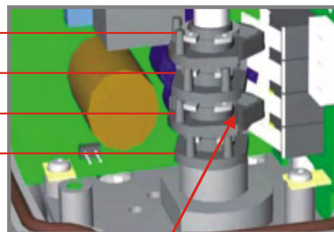
2 mm Inbusschlüssel ansetzen um Nocken zu verstellen.
