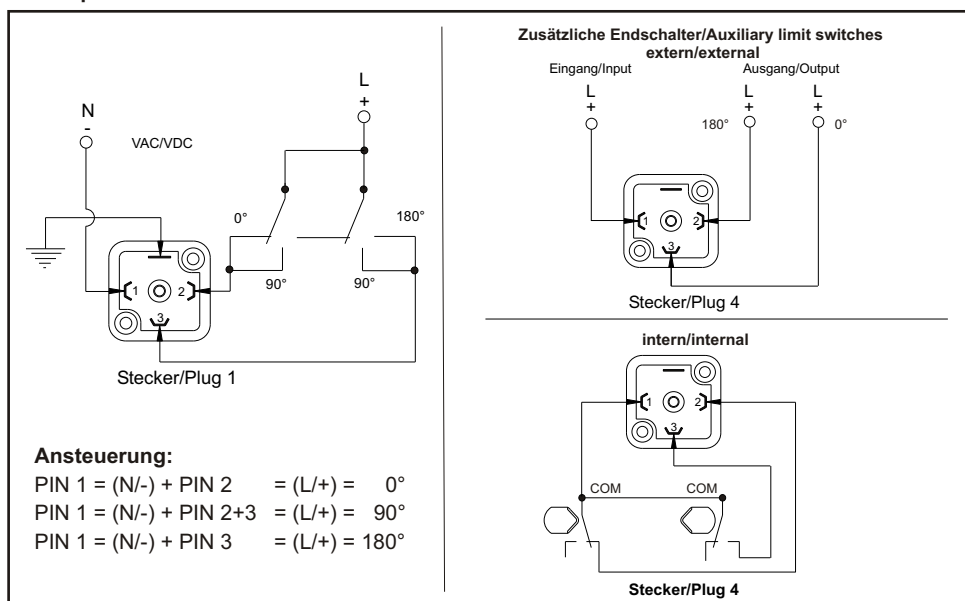
Schaltplan für EJ3 / EJ3C Modelle 0° - 90° - 180°
