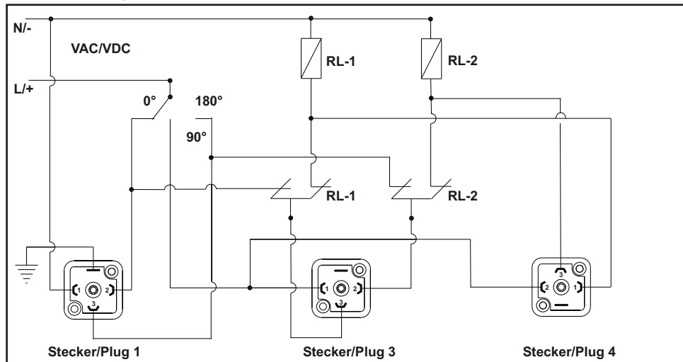
Standardschaltplan für EJ2 Modelle - 0° - 90° - 100°
