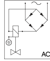
Anschlussplan / Connection diagram
